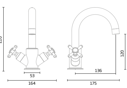
Chrome -TR1070
