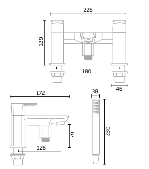
Chrome -TR1055
