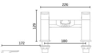
Chrome -TR1053
