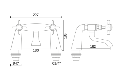
Chrome -TR1057
