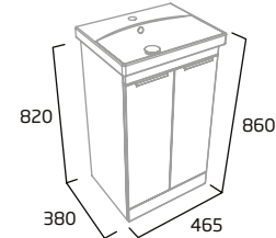
500mm Freestanding 2 Door Wash Unit
