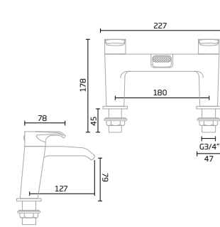
Chrome -TR1043
