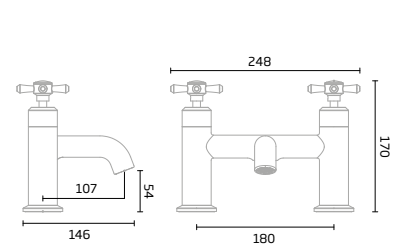
Chrome -TR1071
