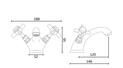
Chrome -TR1056
