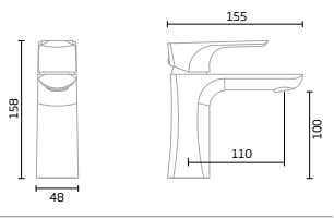
Chrome -TR1061
