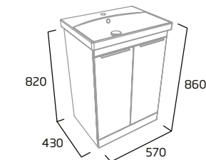
600mm Freestanding 2 Door Wash Unit
