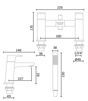
Chrome -TR1038
