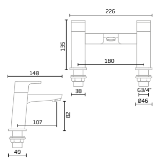
Chrome -TR1037
