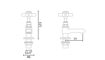
Chrome -TR1059
